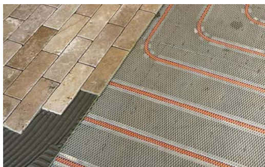
Exemple de pose directe de carrelage sur l'émetteur avec du mortier-colle flexible.
